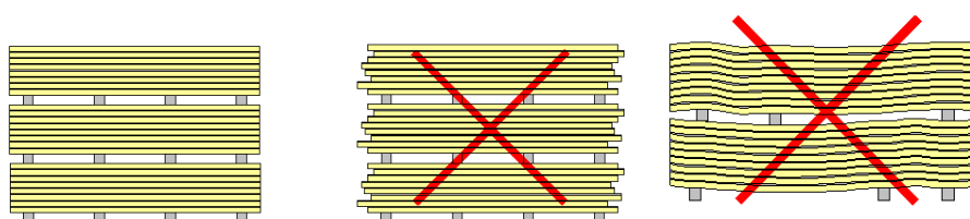
Рис. 1. Розташування ЛДСП під час зберігання
