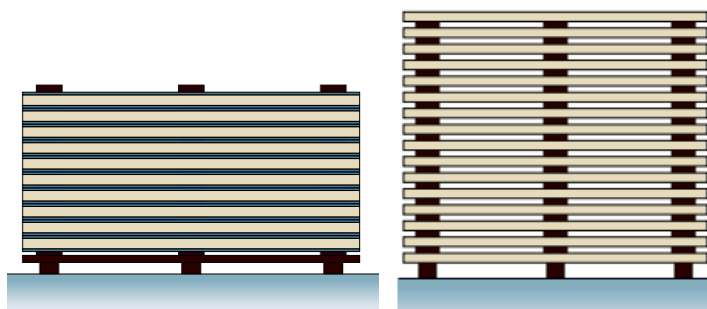
Рис. 5. Акліматизація ЛДСП
